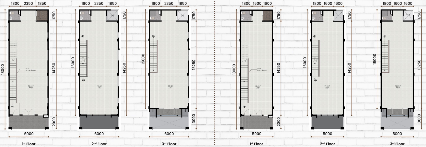
Standard Type 6 x 18 LT : 108 m 2 | LB : 282 m 2
